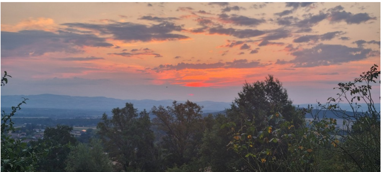
Схід сонця з Марсілли-ле-Шатель (Франція) у напрямку Носівки (Україна)
